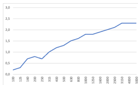
Prova effettuata su pannelli non in aderenza (montaggio tipo J). Valori riferiti alla misurazione sulla singola unità di dimensioni 120x120 cm (Superficie esposta 2,88 m 2 ).
