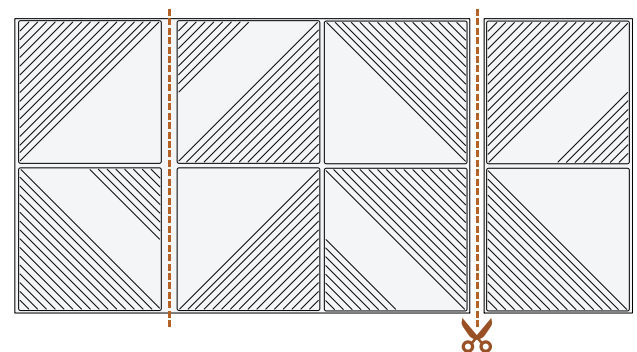
2 moduli doppi 60x120 cm + 1 modulo quadruplo 120x120 cm
