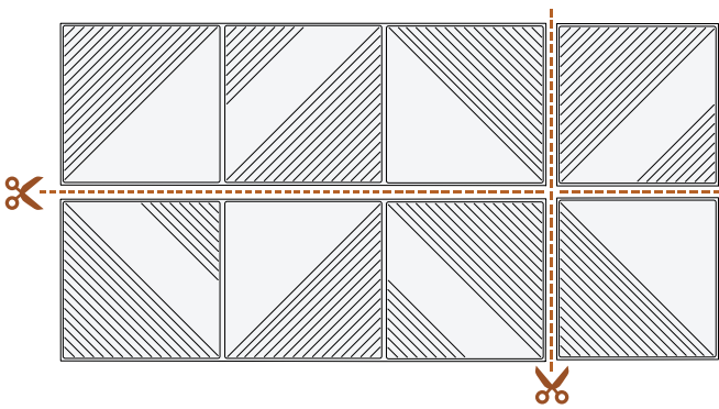
2 moduli tripli 180x60 cm + 2 moduli singoli 60x60 cm
