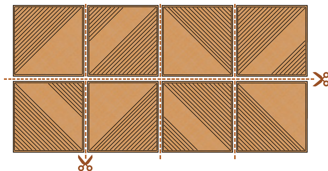
8 moduli singoli 60x60 cm - Colore Giraffe
