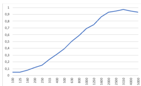
Prova effettuata su pannelli in aderenza al supporto (montaggio tipo A).
